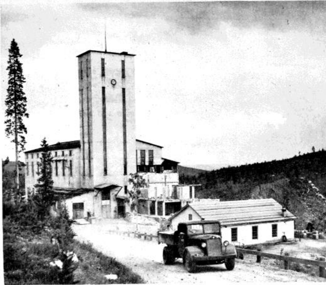
Denna Laver-byggnad är unik inom Boliden-bolaget så till vida att den innehöll alla behövliga utrymmen för gruvdriften — uppfordringslag med bergs- och personspel, krossverk, kul-kvarn, anrikningsverk, kompressorer, el-verk, personalrum, kontor, laboratorium m. m., m. m.
